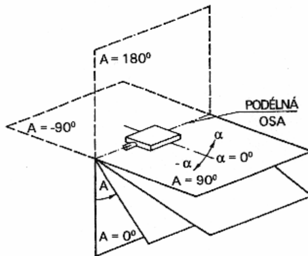
Obr. 2.12 Soustava fotometrických polorovin systému A-a
