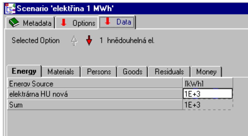
obrázek 7.5 Karta Data pro definování nebo editaci scénářů typu A/B.
