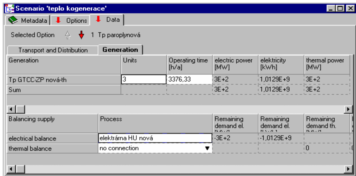
obrázek 7.6 Karta Data pro definování nebo editaci energetických scénářů (Energy only).
