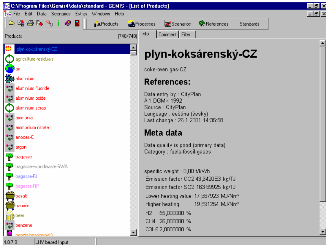
obrázek 7.2 List produktů GEMIS 4.1.
