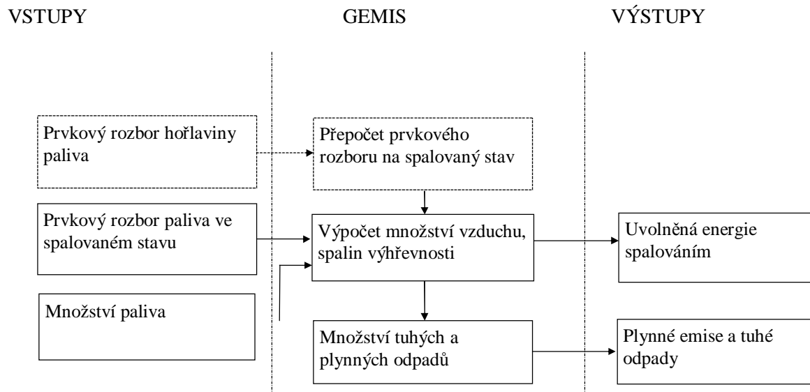
obrázek 5 Schéma výpočtu procesu spalování
