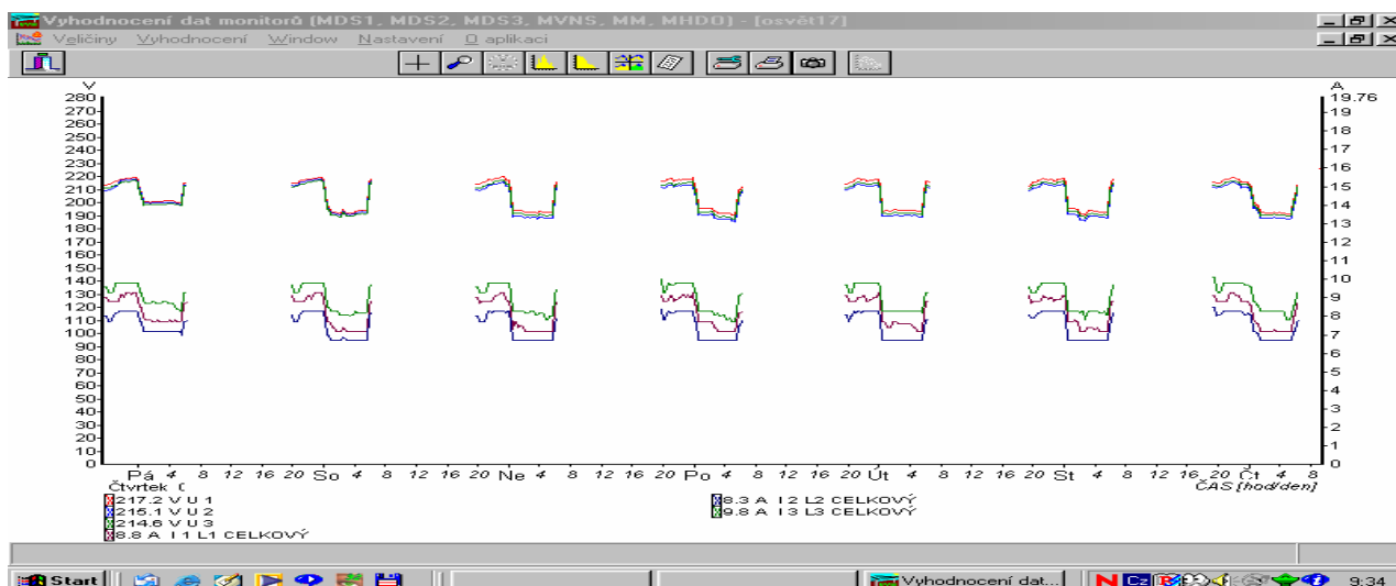
Obr. 5.12 Záznam proudů a napětí při stmívání během týdne
