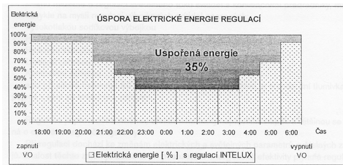
Obr. 5.11 Aplikace regulačního systému
