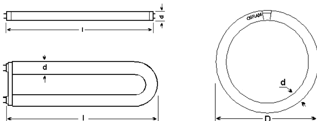
Obr. 2.16 Příklady zářivek
